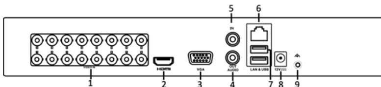
図 1.9DS-7200HGHI-F (/N)
