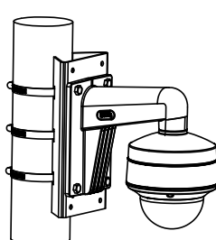
DS-1275ZJ-SUS ポール取付金具
