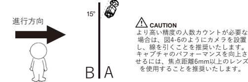
図4-6 人数カウントカメラの設置方法
