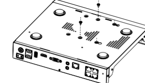
図3-3 ハードディスクの固定
