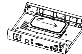
図3-2 ハードディスクの取り付け
