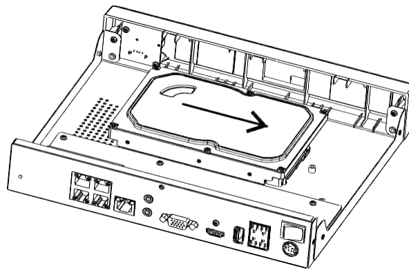
図 3-2 ハードディスクの取り付け
