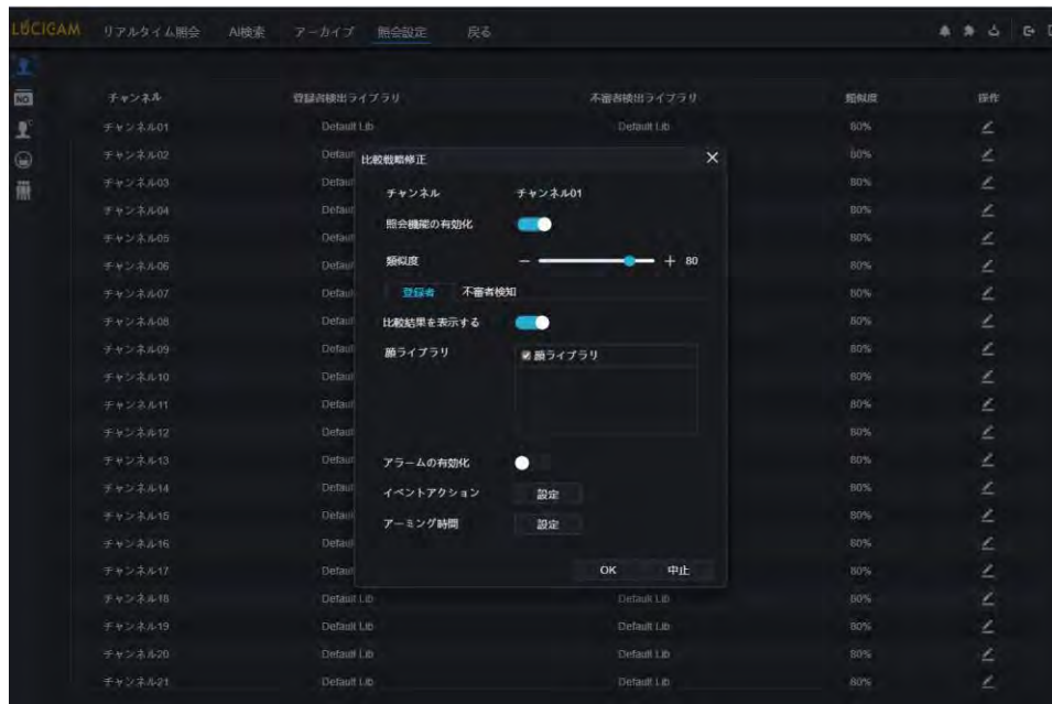
図 8-38 顔比較
