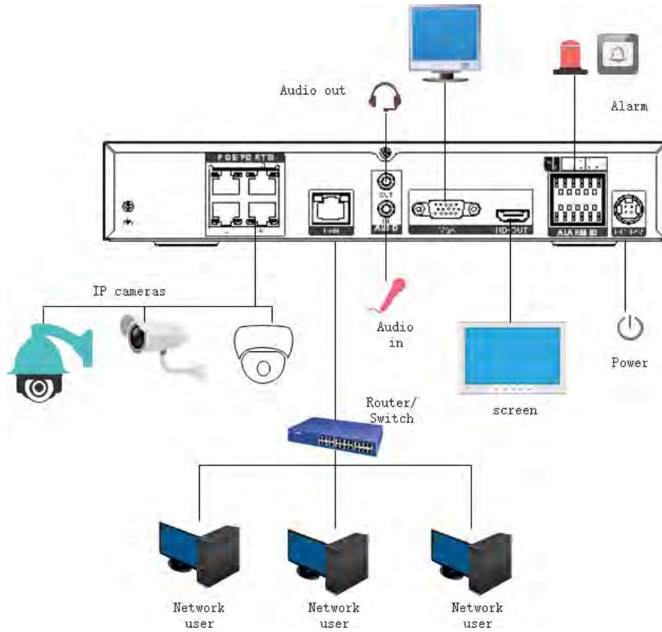
図 2-5 NVRの接続
