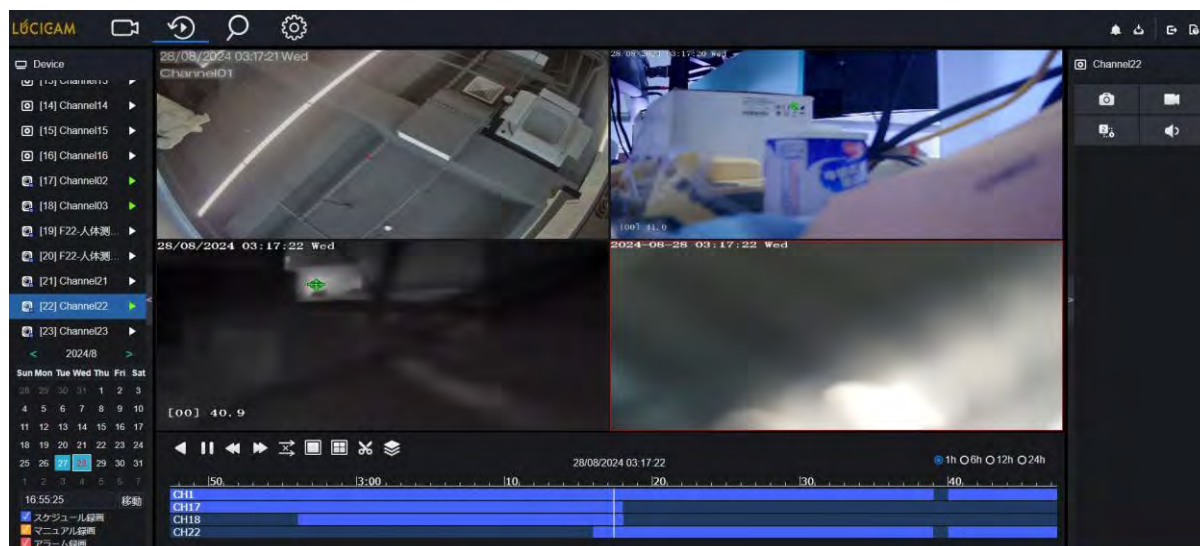
図 8-17 ビデオ再生
